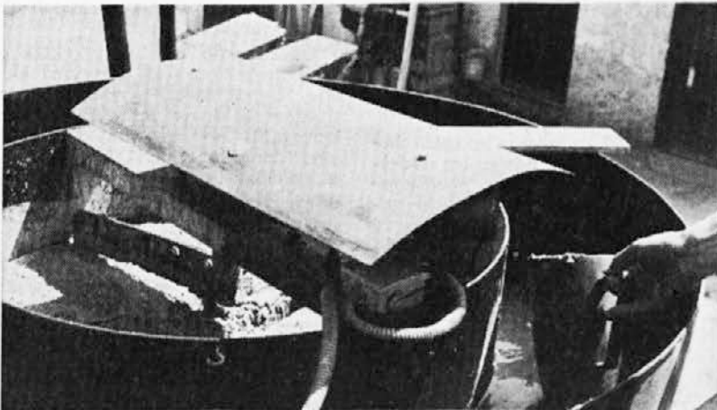
Mulj, ki se je nabral v fluotaciji
