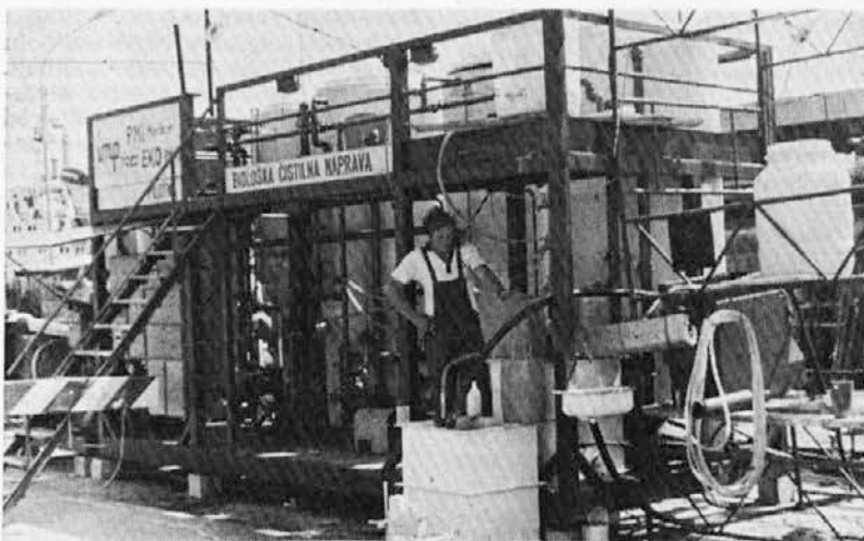
Biolška čistilna naprava
