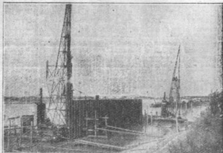
BEOGRAD GRADI PRISTANISCE. Dela so se pričela lansko jesen in zdaj lepo napredujejo. Slika zgoraj: Tako zabijajo Larsenove profile v pristanišču. Slika spodaj: Pogled na sedanja dela ob ustju Save pod Beogradom
