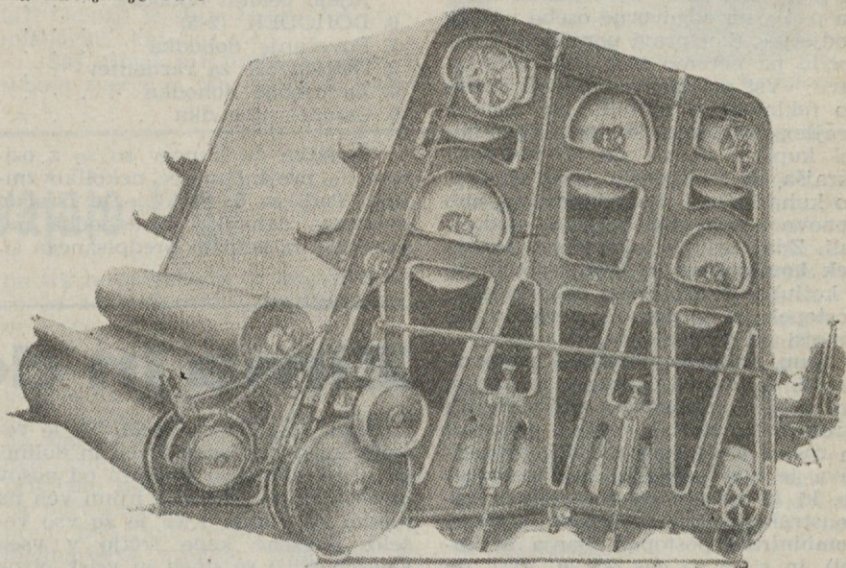
Stari mikalnik z bobnom za navijanje vate
