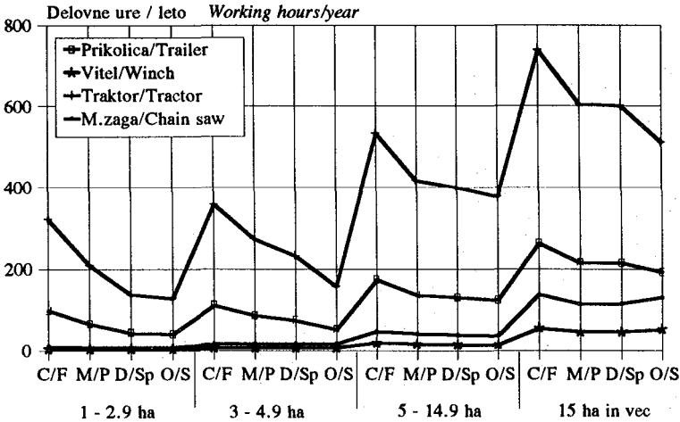
Grafikon 3: Letna obremenjenost delovnih sredstev glede na kategorijo lastništva
