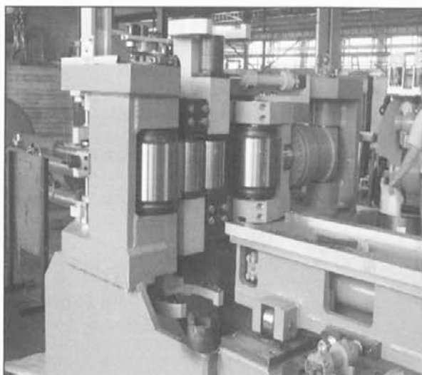
Del linije za valjanje in obdelavo vzmetnih listov
