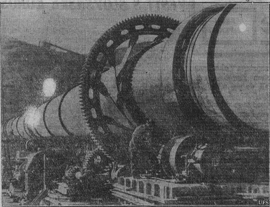
Slika kaže ogromno mašinerijo, postavljeno v Los Altos, Cal., za izdelovanje betona, ki se bo potreboval pri gradbi Shasta nasipa v Central Valley.
