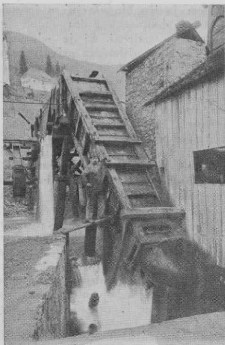
Speljava vodnega pogona valjavnične turbine v Sp. fužini 1876–1908. Ob njem stoji mojster Valentin Šolar, v lini je Janez Lazar. Zidovje stare fužine
