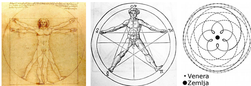
da Vinci: "Vitruvian man"; okultna predstavitev pentagrama; pot Venere okrog Zemlje
