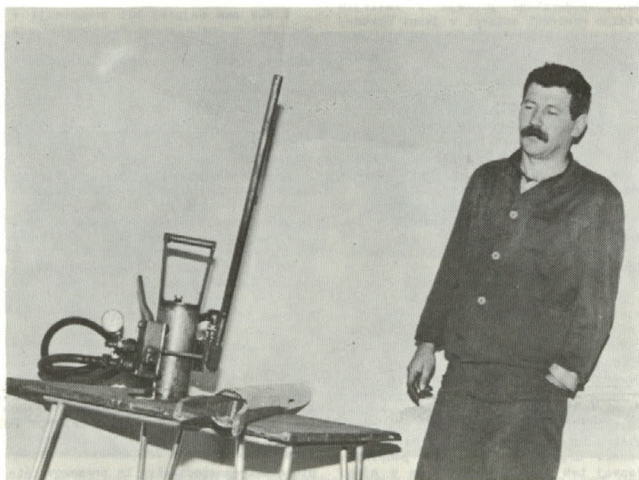
Detektor za ugotavljanje predelov v jami, v katerih so možni nenadni izbruhi plina in premoga, in njem sodelavec inženirja Mayerja Bogo Čurči.
