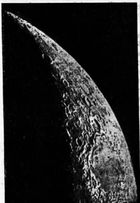
Prvi krajec 3½ dni po mlaju, kakor ga vidimo skozi daljnogled
