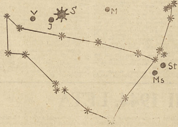
Sonce pred ozvezdjem Kozoroga; zraven njega sta Venera in Jupiter, desno zgoraj Merkur, na desni Mars in Saturn. S — Sonce, J — Jupiter, M — Merkur, Ms — Mars, St — Saturn
