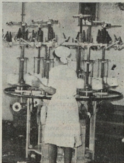
Dosti skrbi povzročajo pletilkam pletilni stroji
