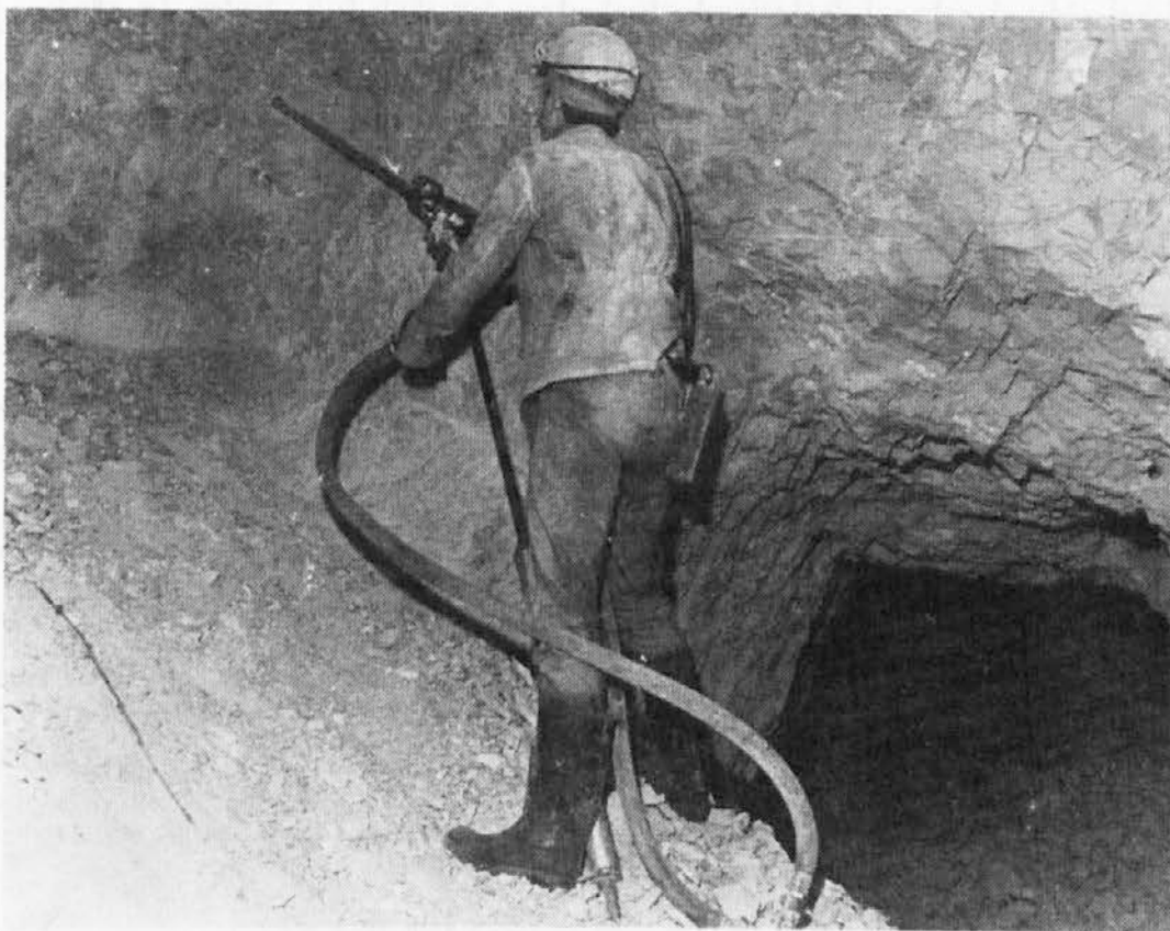
Praktični pouk v jami
