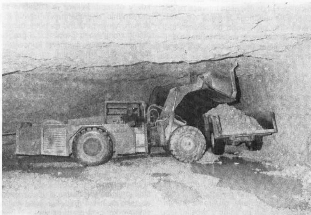
Nakladalni stroj in kamion na gumijastih kolesih sta velika sprememba za jamsko tehniko. Vrtalnega stroja, ki spada v garnituro, še ni.
