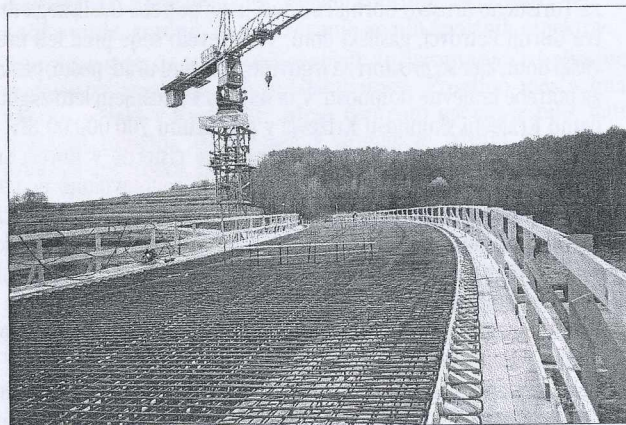
Izgradnja nadvoza N7 na cesti G. Petrovci - Križevci
