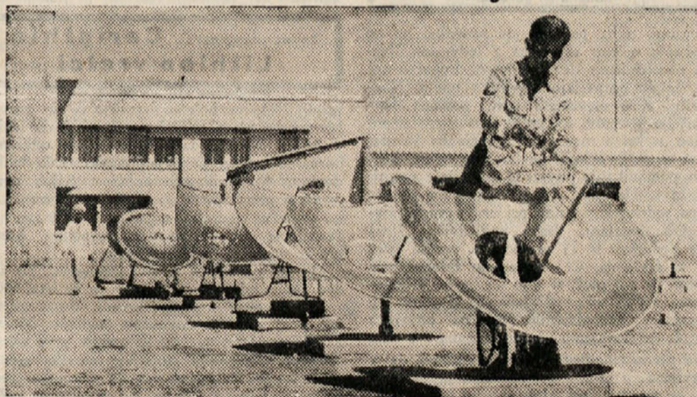
Britanski znanstvenik A. L. Gardner, ki živi kot svetovalec UNESCO v Indiji, je prišel na idejo, da bi se tam dala ekonomsko izkoristiti jakost sončnih žarkov. Izdelal je načrt posebnega kuhalnika, ki izkorišča sončno energijo. Take sončne kuhalnike kaže naša slika na neki razstavi v New Delhiju. Pravijo, da indijski ministrski predsednik Nehru že uporablja tak sončni kuhalik. (AND)
