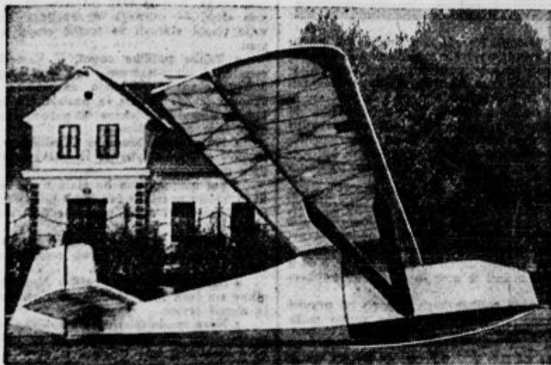
Vadniška jadrilica »Inka«, prva slovenska konstrukcija.
