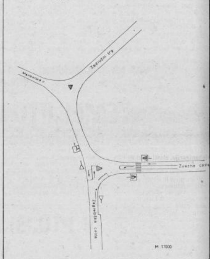
Ureditev prometa v križišču magistralne ceste M/3 in Zagrebške ceste Ptuj (Besedilo je že na skici!)
