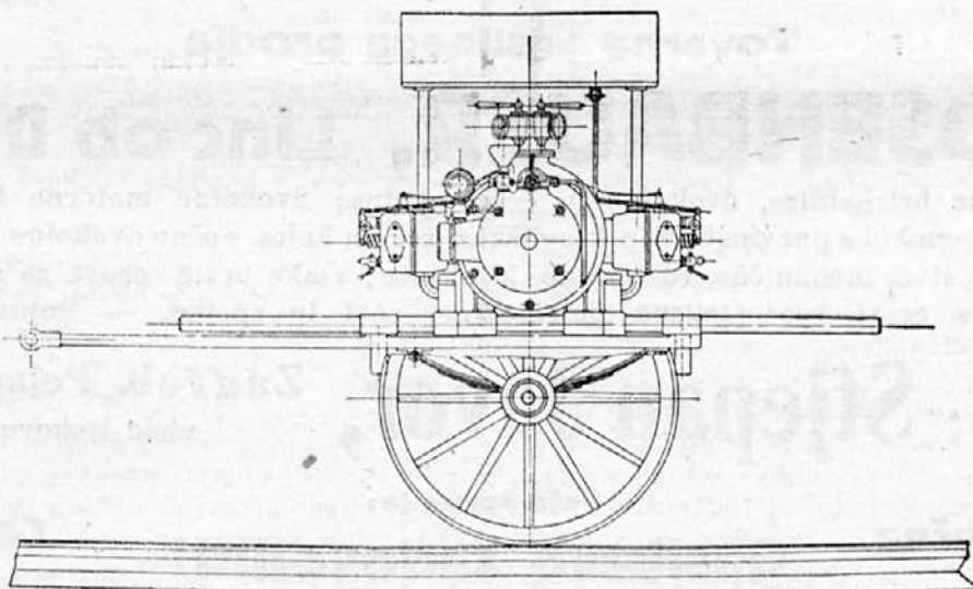
Dvokolna snemalna motorna brizgalnica
