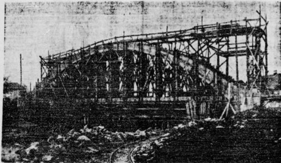
Banovina je zgradila pri Podpeči nov železobetonski most čez Ljubljanico, ki je veljal 1.150.000 Din.
