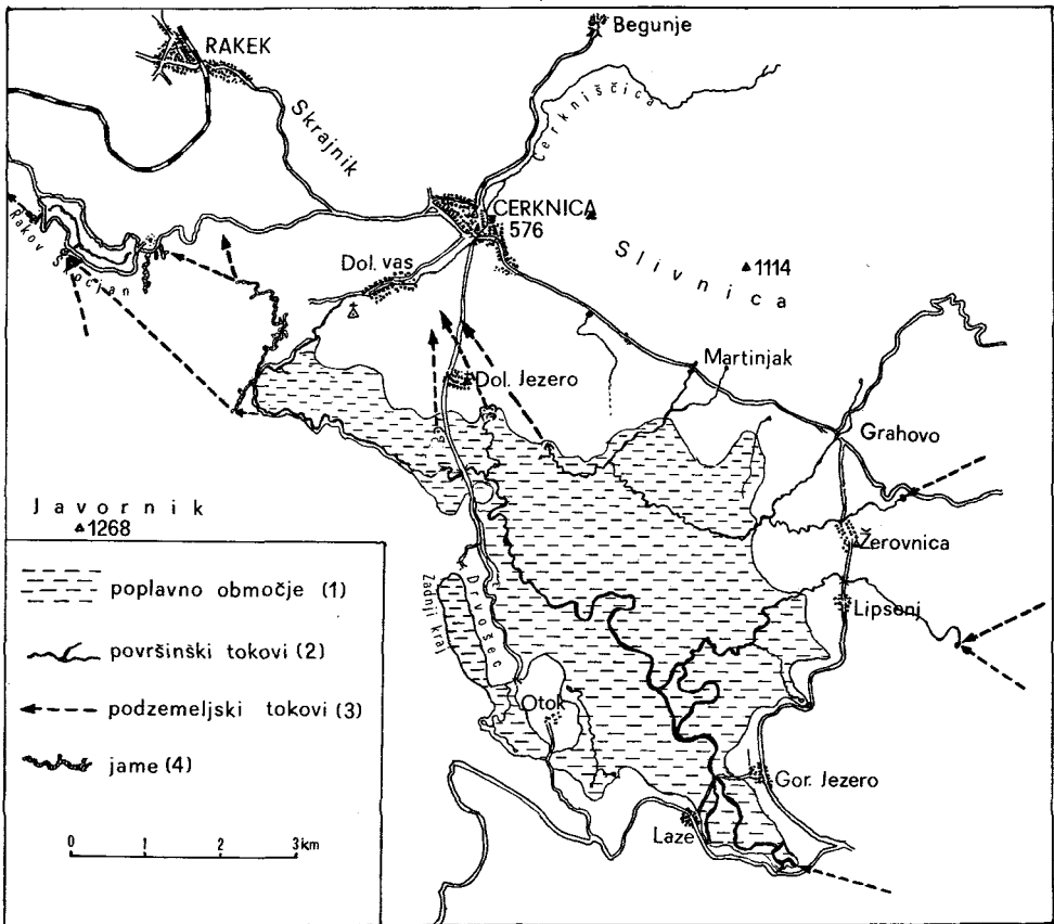
Sl. 1. Hidrografske razmere Cerkniškega jezera in okolice: poplavno območje (1), nadzemski tokovi (2), podzemski tokovi (3), jame (4)
