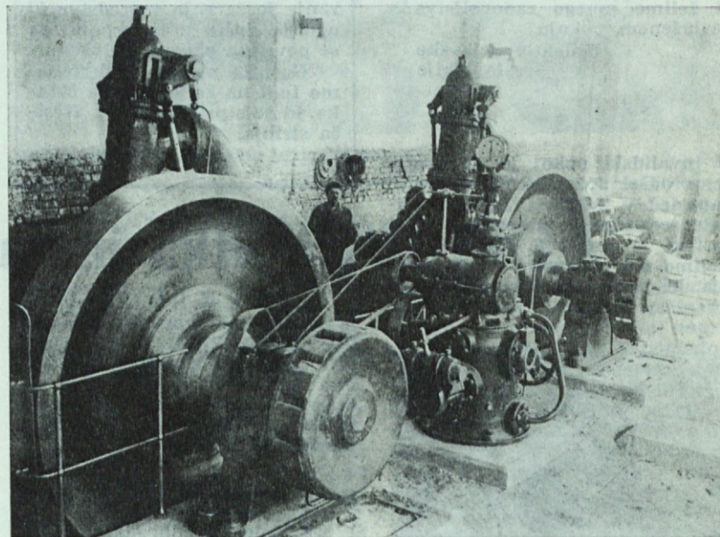
Orumenela slika HE Završnice iz albuma gospoda Slovnik iz Sydneya
