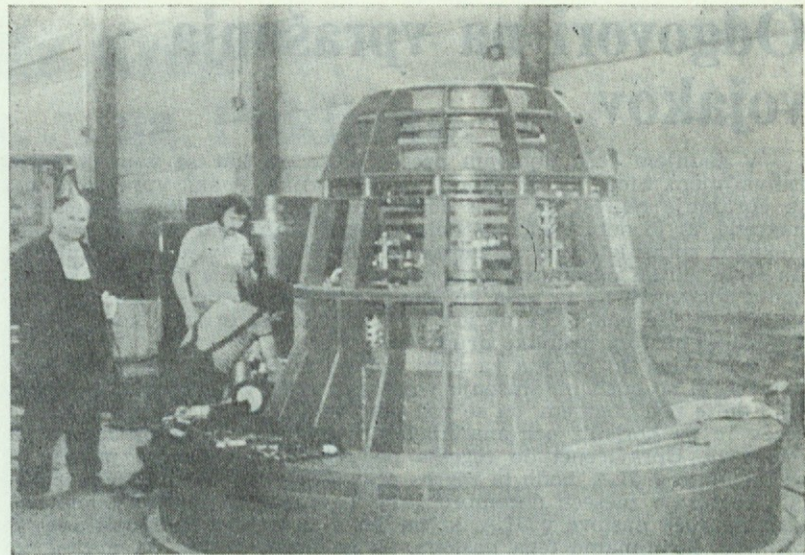
Cabra Corral — turbina »A« pred zagonom
