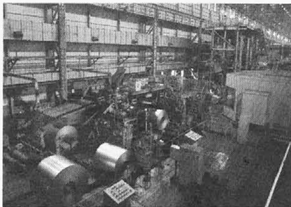
Notranjost hladne valjarne v Posci, ki so ji Stroj Ravne, d. o. o. lani prodali prvih 12 pogonskih in delovnih valjev
