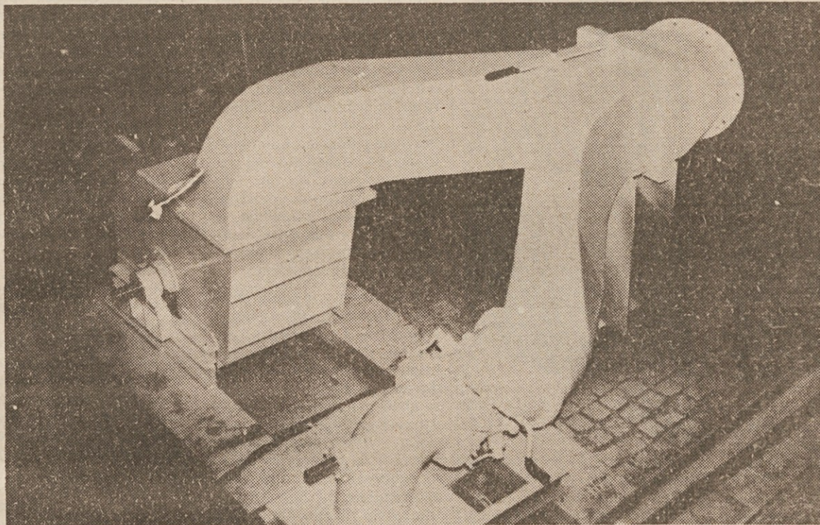
Cevna in Bankijeva turbina za pretočno hidroelektrarno v Polšniku.
