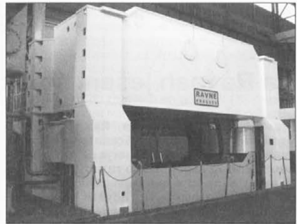
3000-tonska stiskalnica za podjetje Fapco iz Detroita je imela večjo silo na prvi polovici paha.
