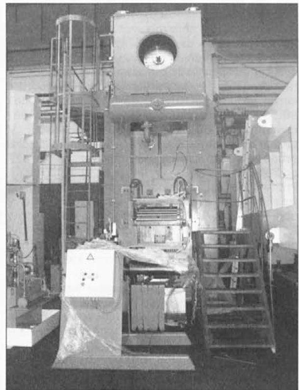
Stiskalnica s spremenljivim gibom hoda s podajno linijo za podjetje Schmittenberg, izdelana poleti 2006.
