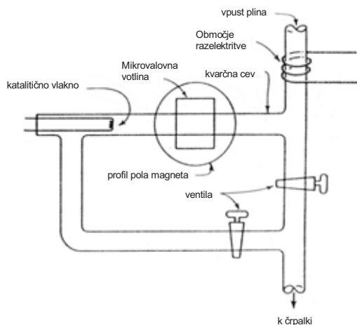
Slika 3: Shema postavitve eksperimenta za določanje gostote atomov z EPR. V mikrovvalovni votlini z elektronsko paramagnetno resonanco določijo gostoto vodikovih atomov, ki se nato rekombinirajo na katalitičnem vlaknu
