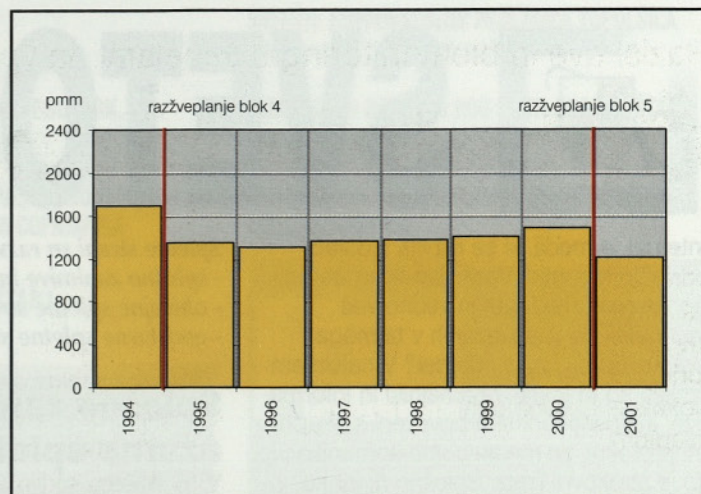
Slika 4: Vsebnost žvepla v tekočih letnikih smrekovih iglic.
