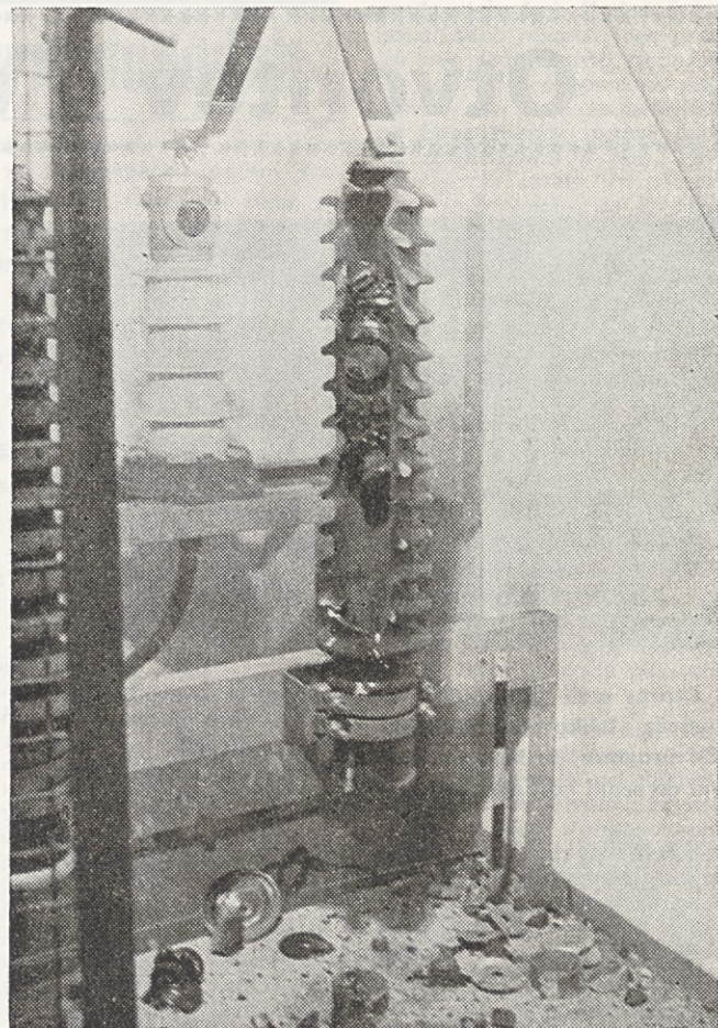
Okvara katodnega odvodnika na transformatorski postaji III je zahtevala 2 uri prekinitve električne napetosti, in s tem tudi dela (na sliki pokvarjeni katodni odvodnik)
