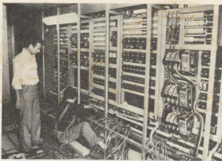
Energetska omara med montažo
