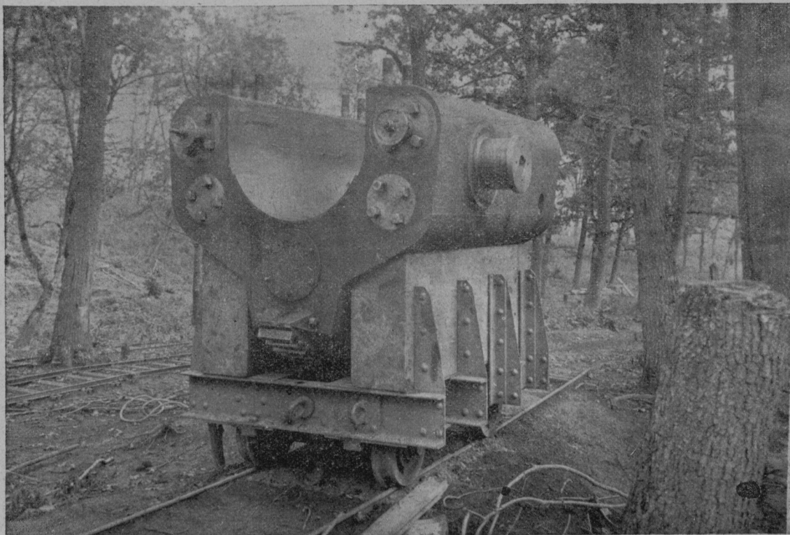
Ruski možnar na kolesih: Pri zadnji ruski ofenzivi so uporabljali Rusi ta ameriški fabrikat. Pri Krivem blizu Břežan je ostala polovica možnarja.
