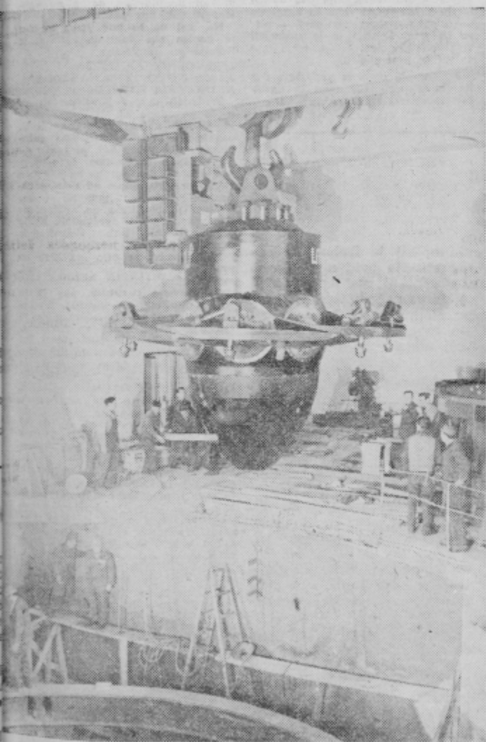
Zerjav Metalne je pričel 120-tonsko breme počasi spuščati v turbinski jašek (Foto: D. Skofič)
