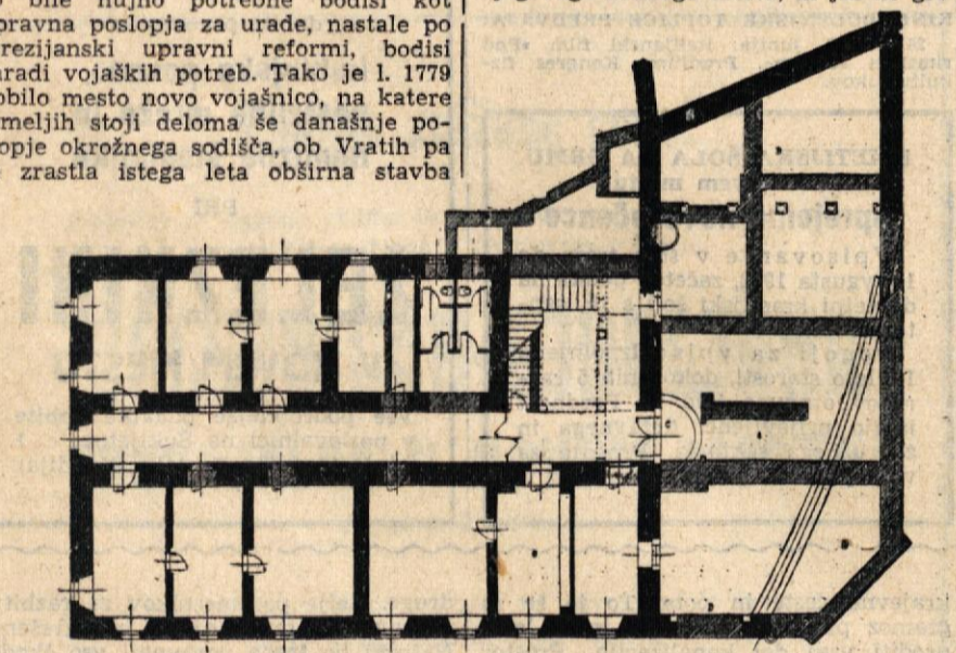
Tloris Kresije z novo ureditvijo trga pred njo: (Risano po načrtih arch. M. Mušiča) Poševno črtkanji zidovi se porušijo. A: no vi trg, B: lopa na stebrih, C: vhodni portal, D: portal iz Soteske, E: novo cestnišče.
