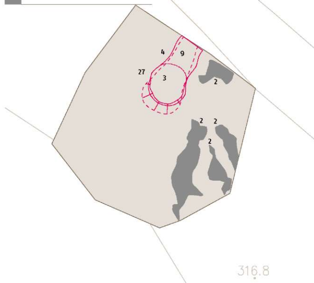
14 Tloris sektorja 4; M 1:100.
