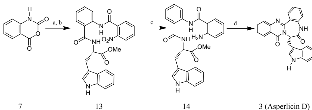
Scheme 3. a) L-tryptophane methyl ester. \text{Et}_3\text{N} , \text{CH}_3\text{CN} ; b) 2\text{-O}_2\text{N-PhCOCl} , \text{Et}_3\text{N} ; c) \text{SnCl}_2\cdot x2\text{H}_2\text{O} , \text{MeOH} , reflux; d) \text{MgCl}_2 , \text{DMF} ,
