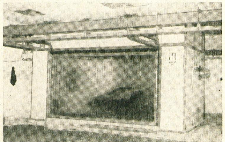
Nova »Pasting« naprava za sušenje usnja, ki so jo uvozili iz Nemčije.
