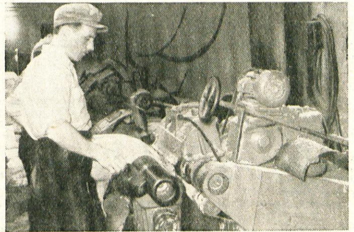
Na brusilnem stroju kože obrusijo, da so enako debele
