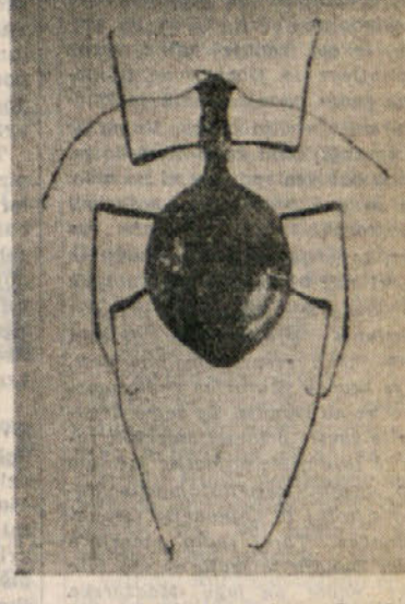
Slepi jamski hrošč-mrhar. Oči bi mu ne služile v temi, zato jih nima; ima pa tembolj razvite tipalke.
