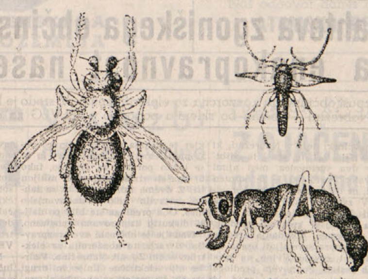
Muhe in metulji iz viharnih otokov Kerguel so brez peruti cili pa imajo te zelo majhne in ne morejo leteti.
