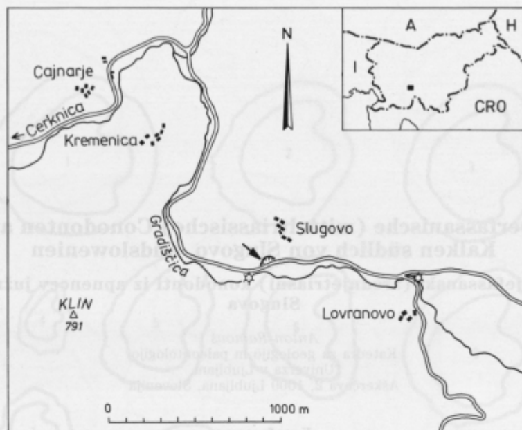
Abb. 1. Lage des Fundortes mit der oberfassanischen Conodontenfauna
