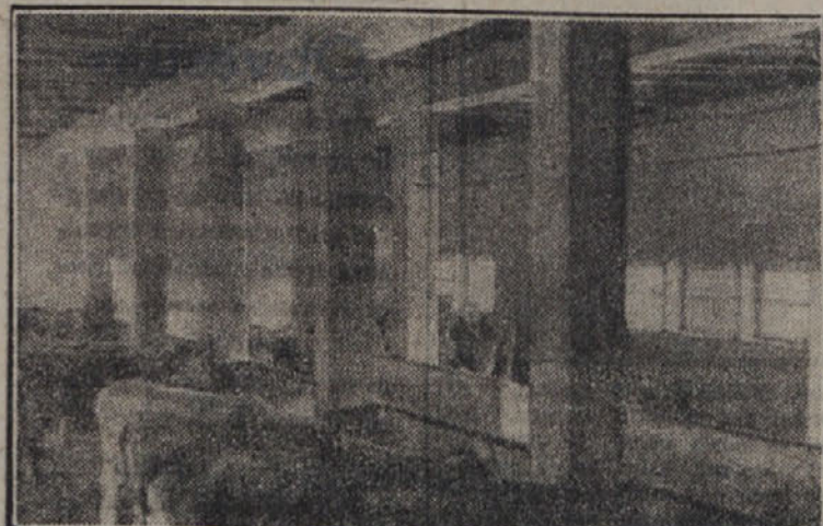
Zadrugni hlev prve obdelovalne zadruge Gabrovice, v katerem stoji 49 glav lepo r ejene živine.
