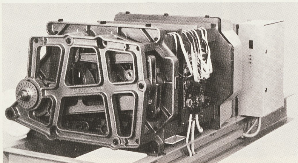
Žakardski stroj CX 860 izrednih hitrosti
