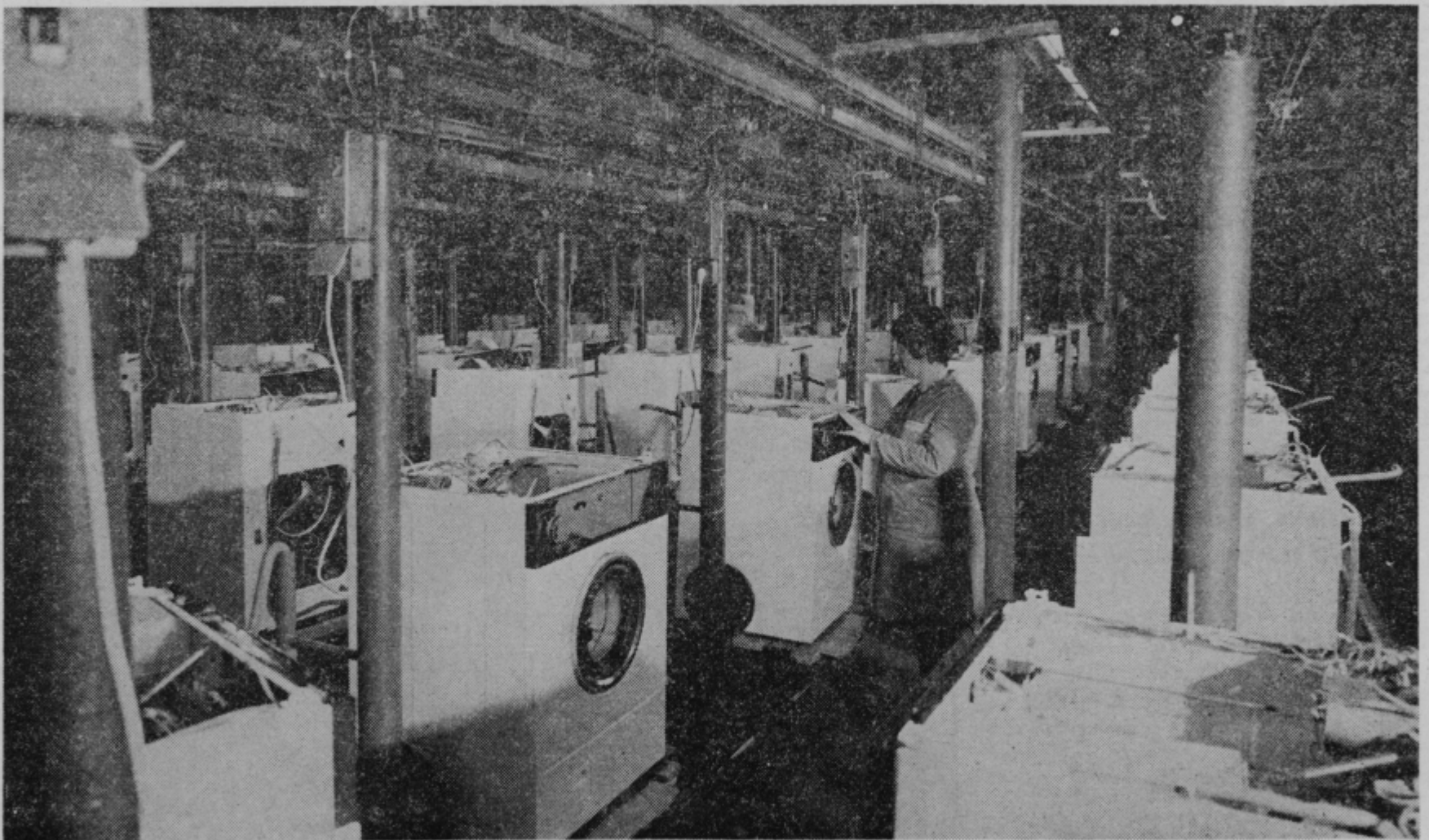
Detajl iz proizvodnje pralnih strojev — ZADNJA KONTROLA V TOVARNI GOSPODINJSKE OPREME
