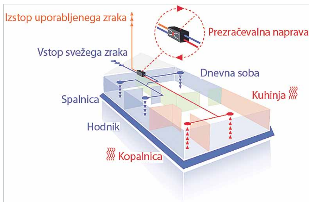
Shematski prikaz prezračevanja z vračanjem toplote
