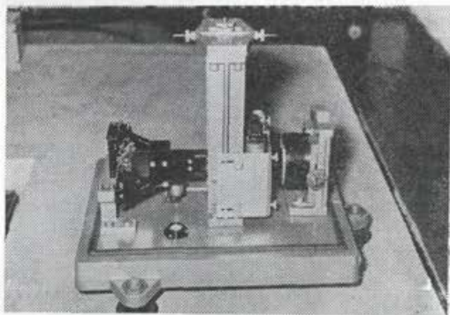
Vertikalni seizmograf Hiller v kleti Astronomsko geofizikalnega observatorija v Ljubljani. Aparat je postavljen na betonskem stebri, ki je ločen od okolišnje stavbe
