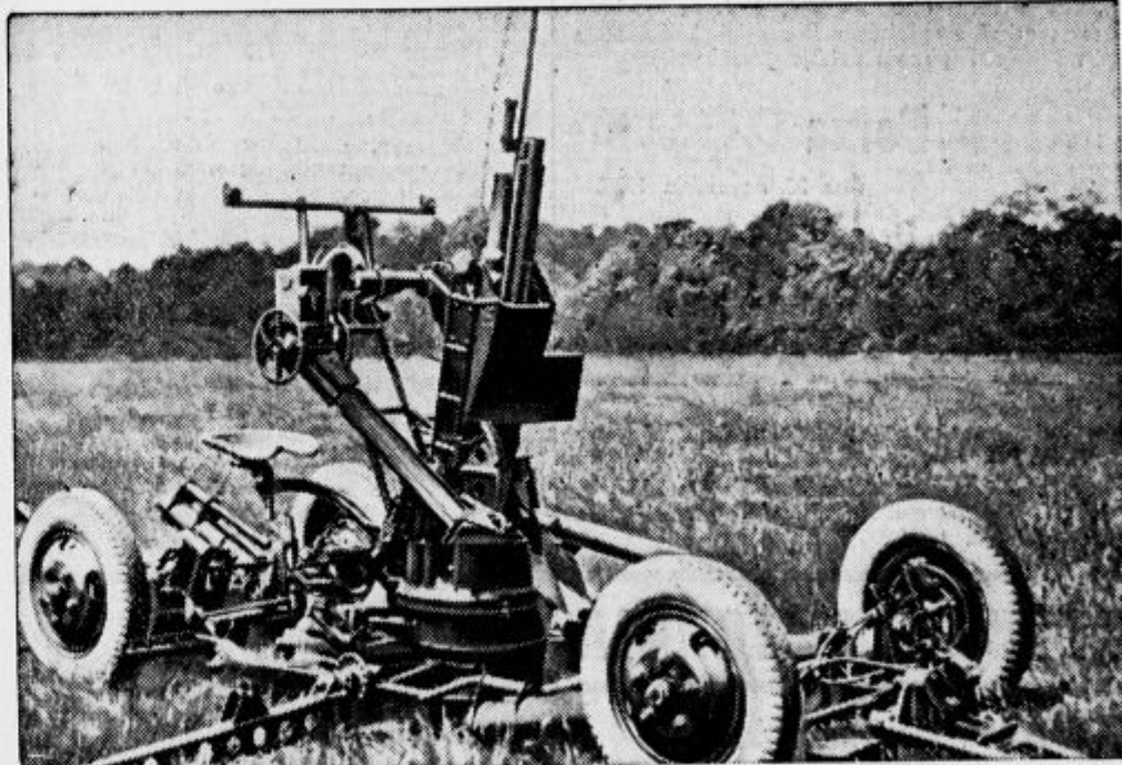
Najnovjši ameriški top za obrambo letalskih napadov Amerika je zgradila nov top proti letalom. Top tehta 5000 funtov in ima kaliber 37-milimetrov
