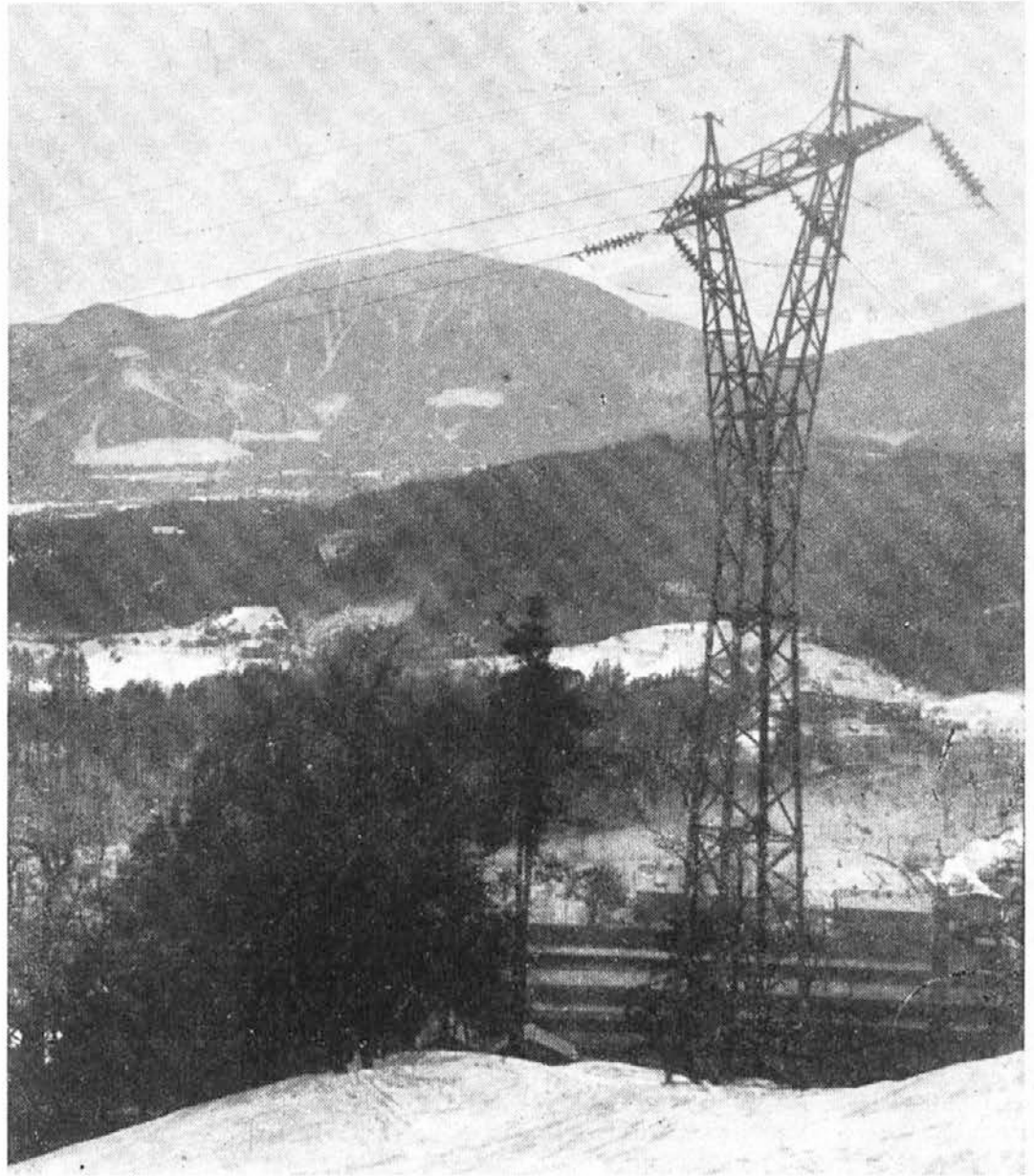
Odlične panorame. Nosilec novega daljnovoda za dovod energije ravenskim fužinam na Tičlerjevem vrhu.
