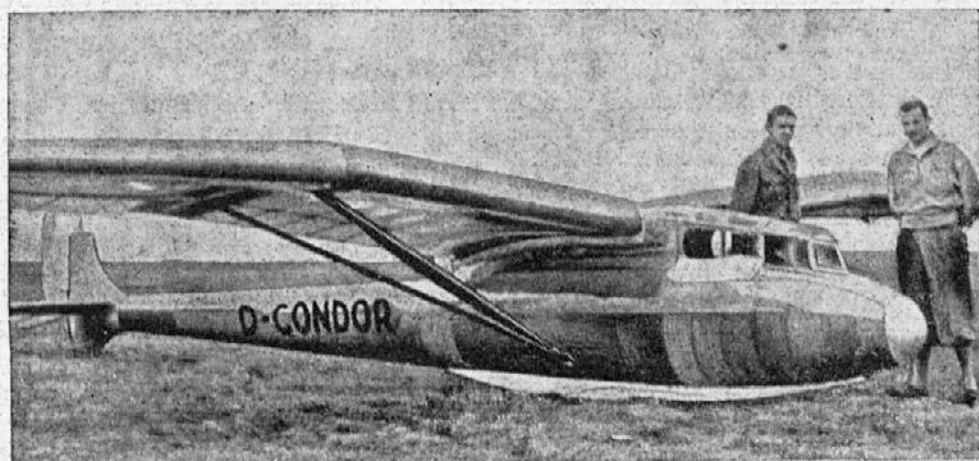
Svetovni rekord z jadralnim letalom. Letalec K. Dittmar s svojim bratom Edgarjem pri letalu, s katerim se je dvignil iz višine 350 m do višine 4200 m.
