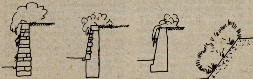
Suhozid Zid iz naravnega kamna Betonski zid Utrditev z grmovjem
