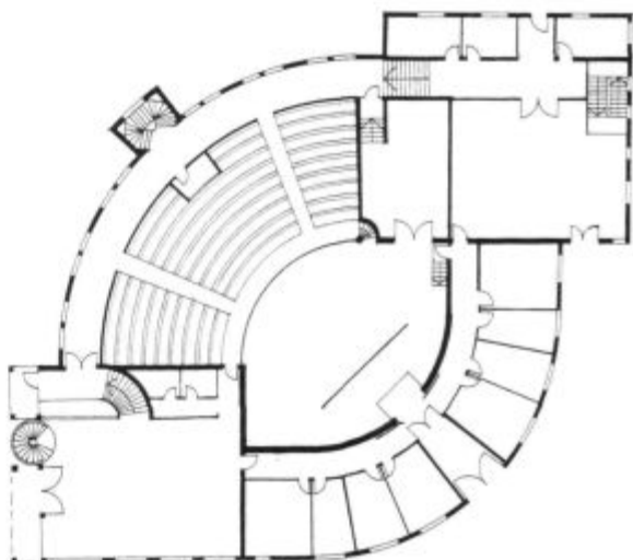
ŠTUDJE FASAD IN PRITLIČNI TLOORIS GLEDALIŠČA
