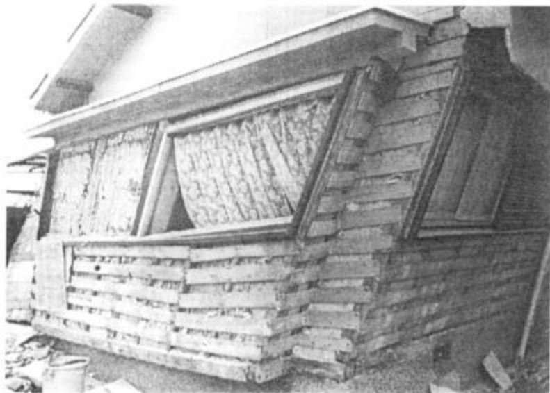
LESENA STAVBA PO POTRESU V KOBEJU. ANALIZA POSLEDIC VELIKEGA HANČINSKEGA POTRESA, DELO, 22. 3. 1995
