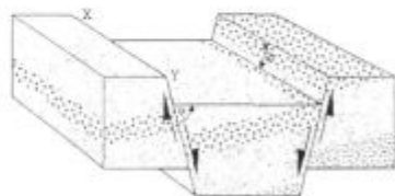
PRELOMNE DEFORMACIJE, GEOLOŠKA PODLAGA IN OBLIKOVANJE POVRŠJA, STR. 15, SKRIPTA SEMINARJA, IDRJA, 1997. (RAZLIČNI VIRI)
