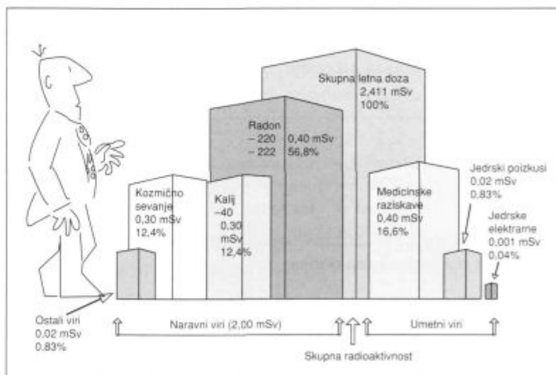
IZPOSTAVLJENOST ČLOVEKA NARAVNEMU IN UMETNEMU SEVANJU NA ZEMLJI.
