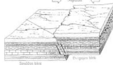
PRELOMNE DEFORMACIJE, GEOLOŠKA PODLAGA IN OBLIKOVANJE POVRŠJA, STR. 15, SKRIPTA SEMINARJA, IDRJA, 1997. (RAZLIČNI VIRI)
