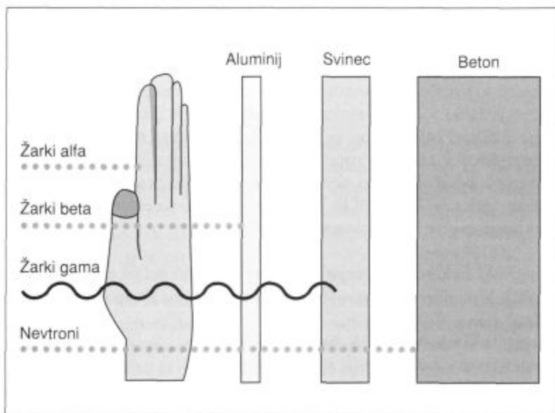
PRODORNA MOČ SEVANJ. NEKATERA ZAUSTAVI ŽE LIST PAPIRJA, DRUGA ŠELE BETONSKI ZID.
