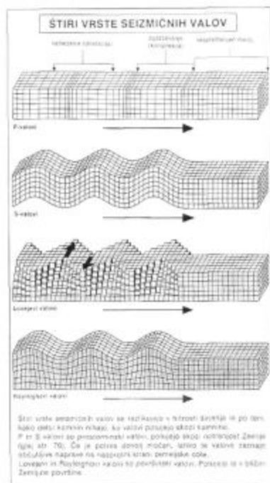
ŠIRJENJE POTRESNIH VALOV, DRUŽINSKA ENCIKLOPEDIJA GUINNESS, STR. 81
