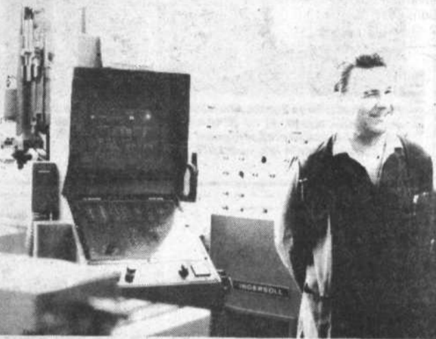
Računalniško voden rezkalni stroj Maho 700, žično-erozijski stroji in programirana miza Fanuc so bistvene pridobitve Tovarne kovinske galanterije, na katere so upravičeno ponosni. Vrednost skupne naložbe je znašala 10,6 milijonov avstrijskih šillingov, z njo pa načrtujejo izvoziti za 5 do 7 milijonov avstrijskih šillingov letno. Trinajst zaposlenih v centru za erodiranje bo, če bo treba, organiziralo delo tudi v treh izmenah. Orodja izdelujejo predvsem iz domačih materialov, le desetina je uvoženih iz sosednje Avstrije. Foto: V. P.
