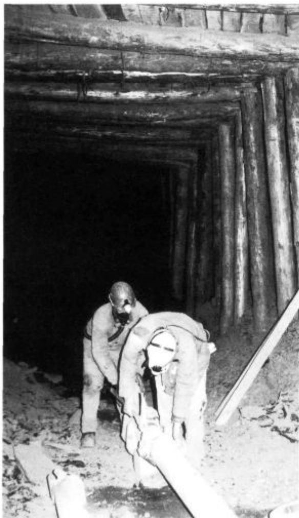
PRIPRAVA ZAPIHOVALNIH CEVI NA ETAŽI KARBON 1/3
