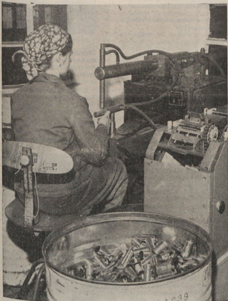
Nova naprava v Izolirki, ki jo spretno upravlja večša delavka, proizvaja pločevinaste tuljce za spajanje bergmanovih cevi
