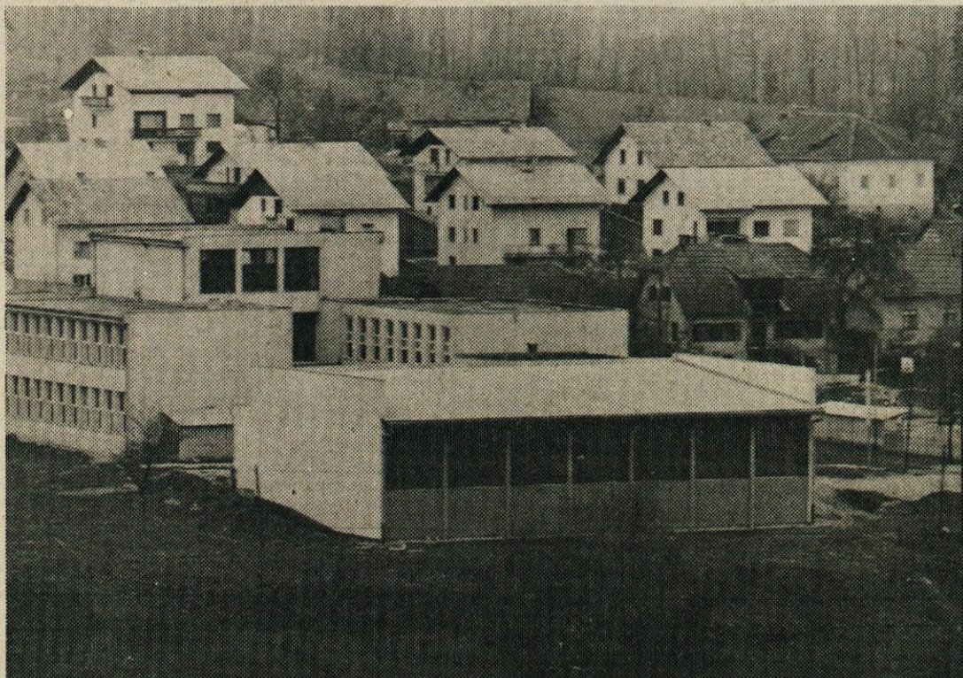
TELOVADNICA PRI OSNOVNI ŠOLIV ŠMARTNEM. Zgrajena je bila januarja leta 1978. Skupna površina je 502 m 2 vrednost del pa 7.173.000 din. V objektu je telovadnica 16 x 28 m, prostor za gledalce (uporaben tudi za tel. vzgojno dejavnost) 6 x 16 m, sanitarije, kabinet in prostor za orodje
